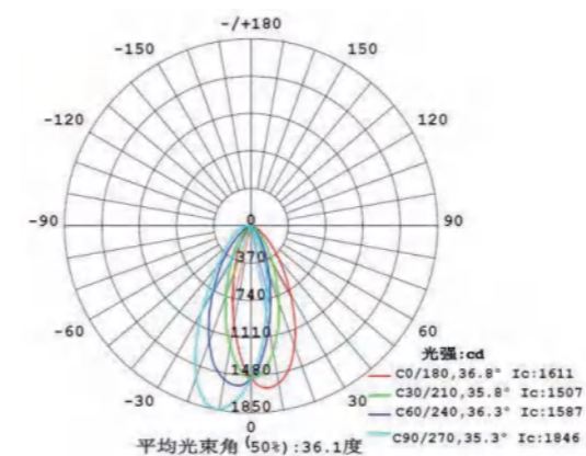
配光曲线
