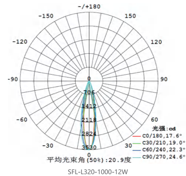
配光曲线
