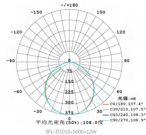
配光曲线
