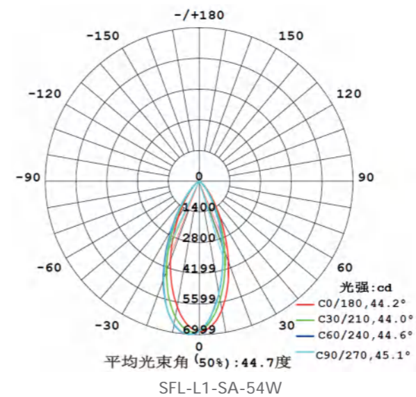
配光曲线
