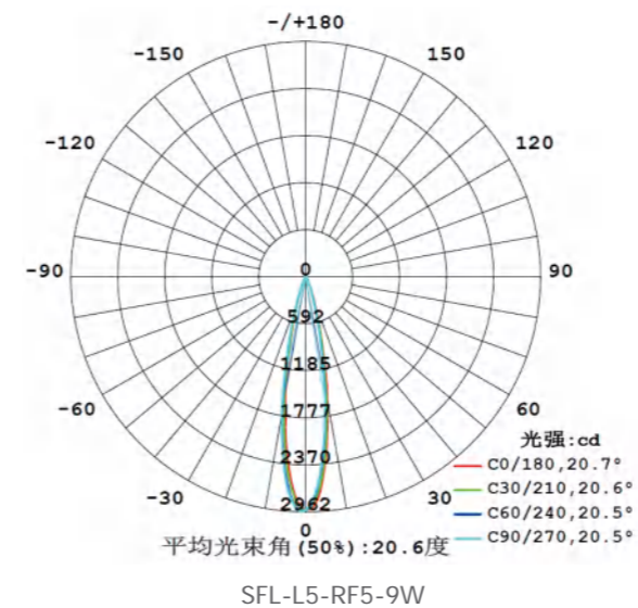
配光曲线
