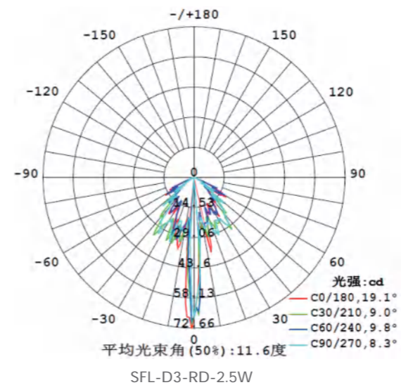
配光曲线
