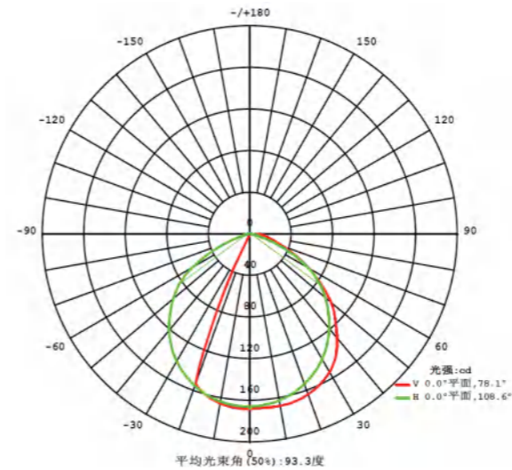
配光曲线
